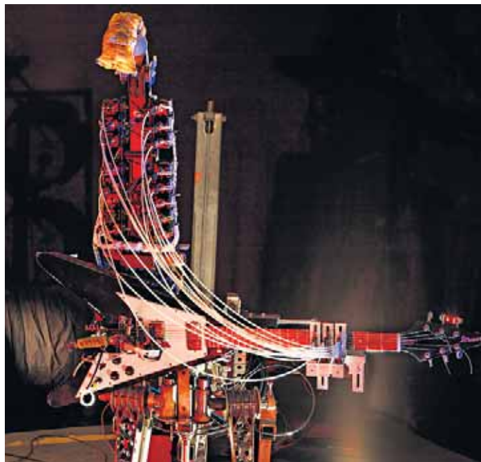
Automatischer Gitarrist: Das Maschinenwesen Lemmi spielt sein Instrument mit 15 Metallfingern.
